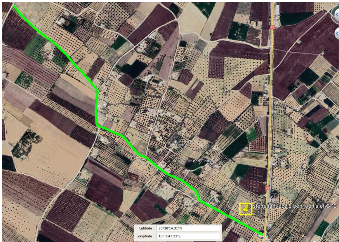
Figure 5: Plan de Piste 05 : Piste reliant ecole beni ounis et GP2
