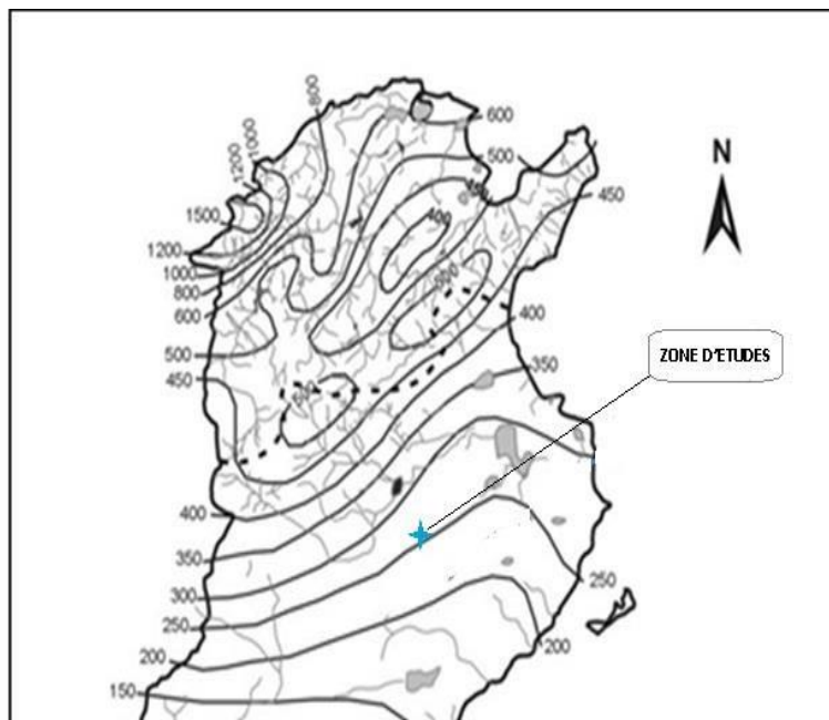
Figure 9 : Carte isohyète
