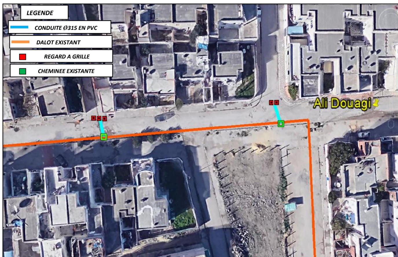
Plan d'intervention Réseau eaux pluviales : Rue ALI DOUAGI
